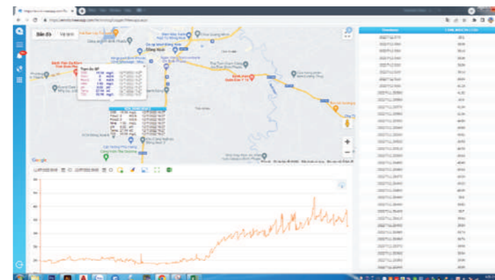
Hình ảnh 1: giám sát thông số Quan trắc nước thải KCN Đồng Xoài III
